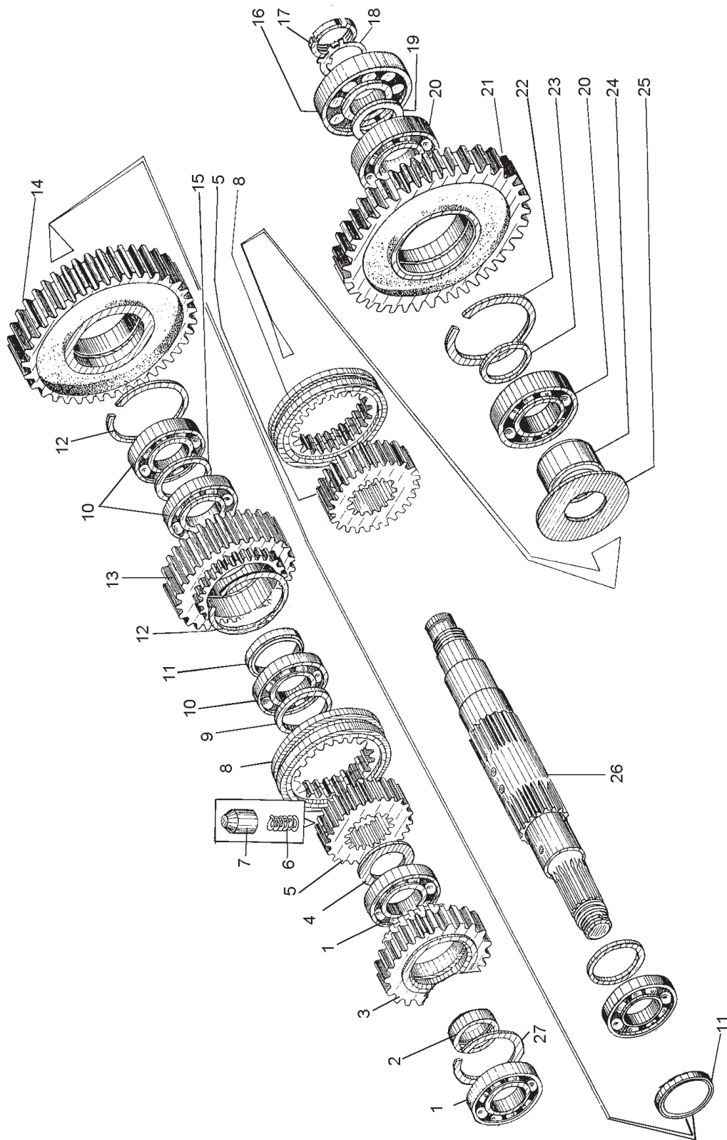
Рис. 4-17 Вал ведущий (ДЗ-98А.10.04.540)
