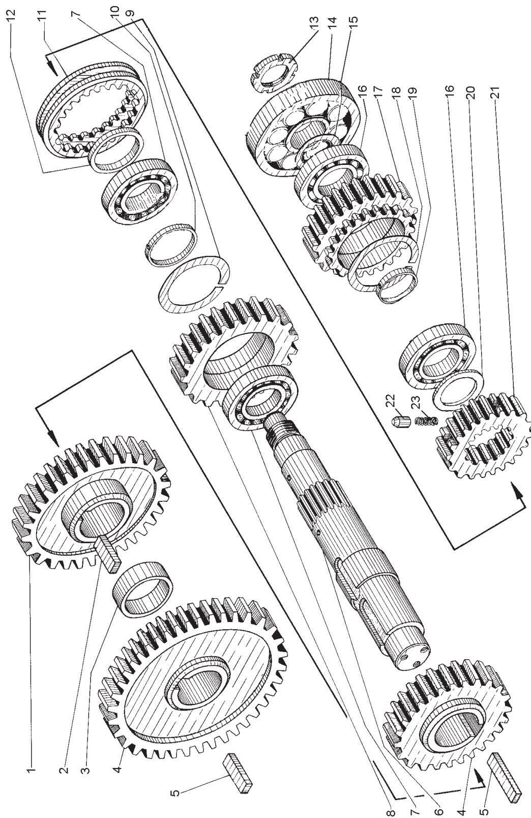
Рис. 4-18 Вал реверса (ДЗ395Б.04.030)
